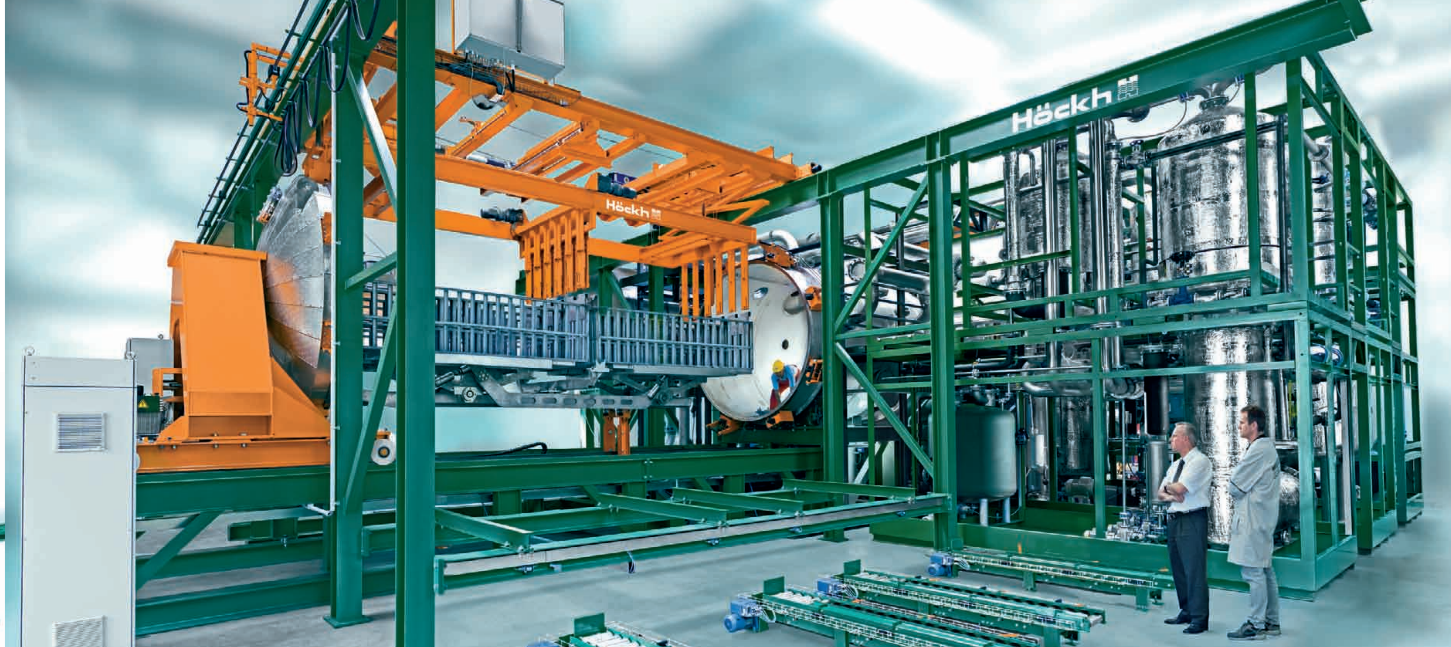
Vakuumanlage Multiclean-6-3-F zur Reinigung von großformatigen Lamellen-Wärmetauschern. Chargenmaß: 6.250 x 1.820 x 1.600 mm. Chargengewicht: 3.500 kg. Lösemittel-Füllvolumen: 60.000 Liter.
